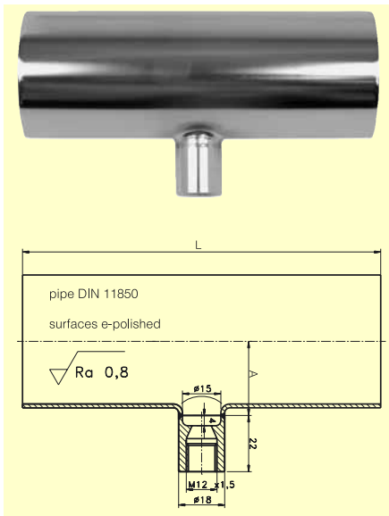
EHG-.../M12 尺寸表
