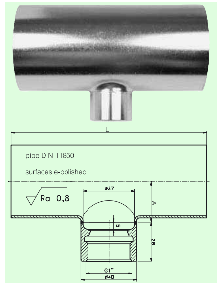
EHG-.../1" 尺寸表
